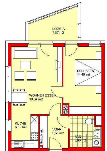
Grundriss Betreubares Wohnen
